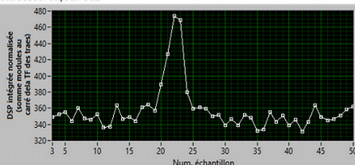
Module de DSP acq Det1-Det2
