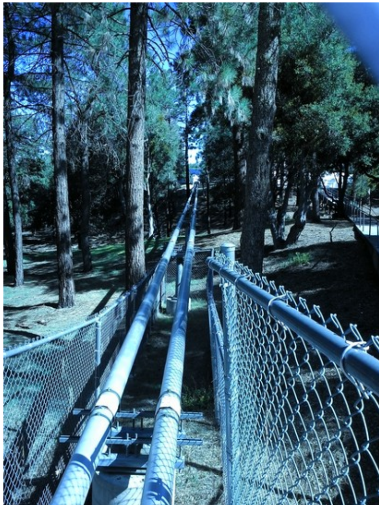
des télescopes vers la station de recombinaison
