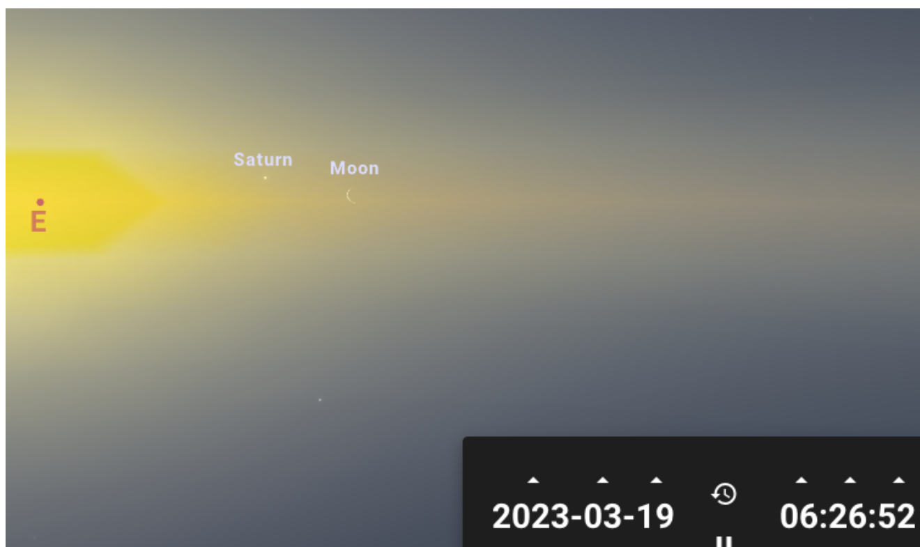
Croissant lunaire et Saturne peu avant l'arrivée du Soleil.
