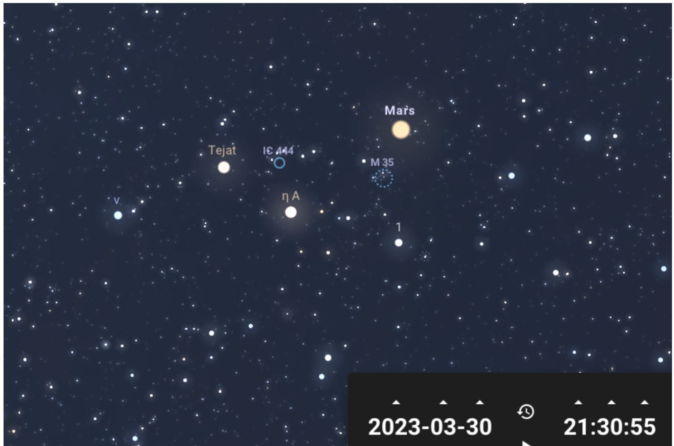
Conjonction entre Mars et M35, dans les Gémeaux, le 30/03/23.
