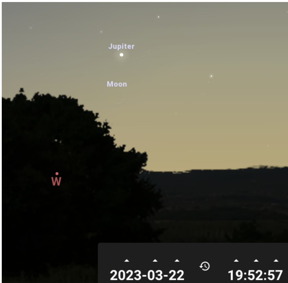
Lune et Jupiter après le coucher du Soleil du 22/03.
